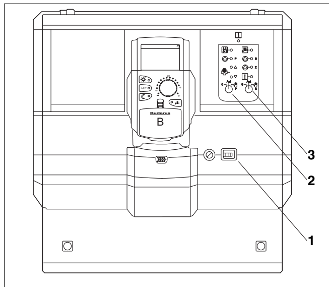
Рис. 17 Logamatic 4126
